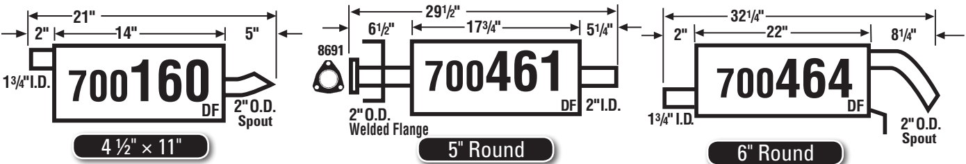
91-02 Sedan, Coupe, Sta. Wag.
