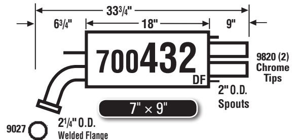
95-96 Camry Coupe, Sedan, 6 cyl.
