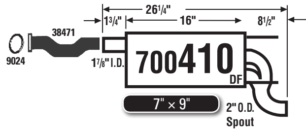
91-93 Accord EX; Sta. Wagon
