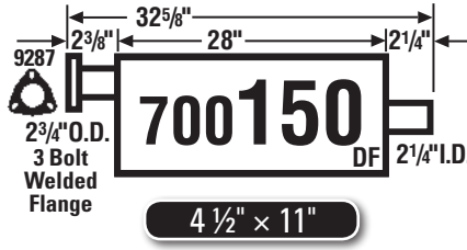
95-99 S10/T10, Blazer/Jimmy, 4-Dr. 96-99 Bravada
