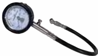
BEP15151 0-15 PSI BEP15152 0-30 PSI BEP15153 0-60 PSI
